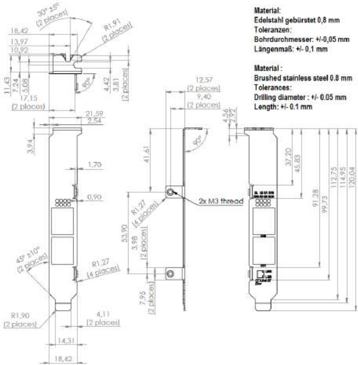
Blenden-Ausschnitt Panel cutout
